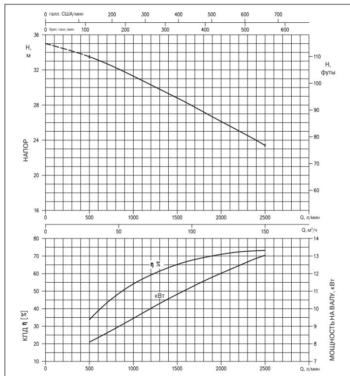
ГРАФИК РАБОЧИХ ХАРАКТЕРИСТИК серии 100DML515 (по ISO 9906, Приложение А) ДИАМЕТР РАБОЧЕГО КОЛЕСА: 309 мм
