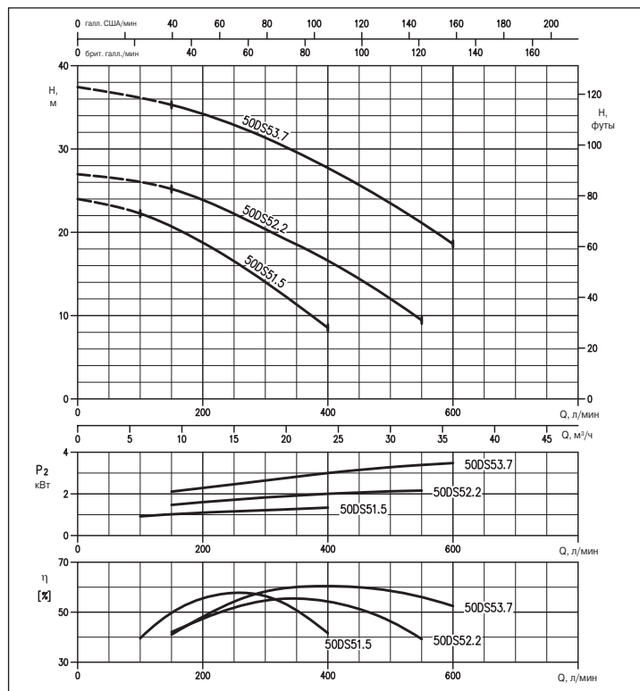
ГРАФИК РАБОЧИХ ХАРАКТЕРИСТИК серия 50DS51.5 (1,5 кВт) серия 50DS52.2 (2,2 кВт) серия 50DS53.7 (3,7 кВт)
