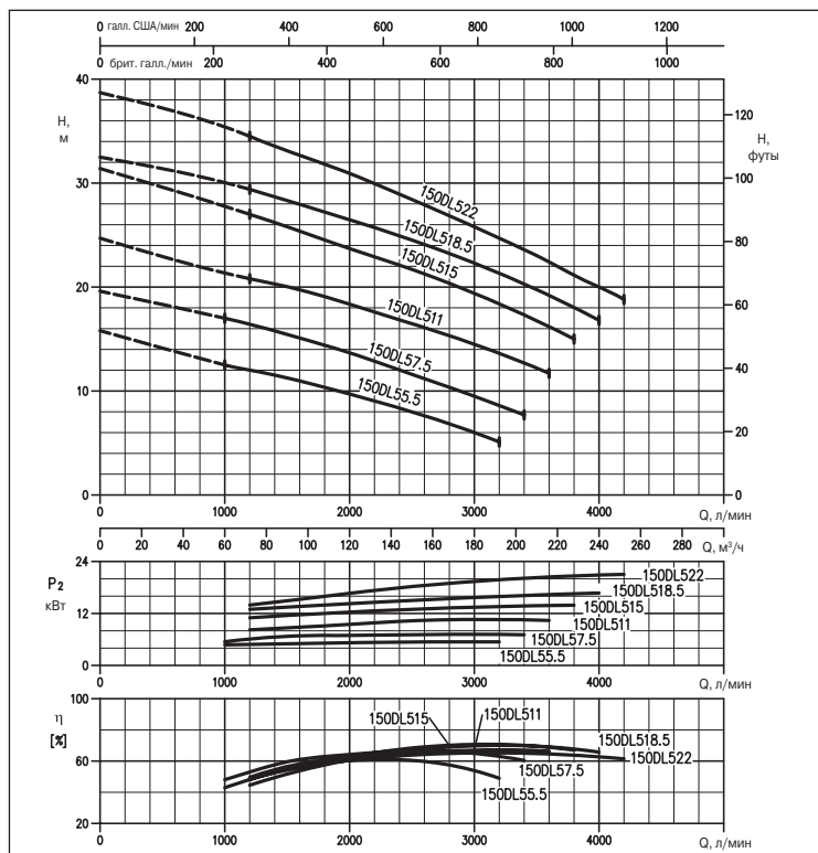
ГРАФИК РАБОЧИХ ХАРАКТЕРИСТИК (по ISO 9906, Приложение А)
