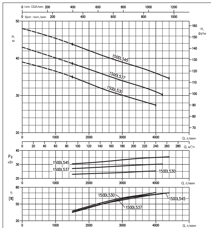
ГРАФИК РАБОЧИХ ХАРАКТЕРИСТИК (по ISO 9906, Приложение А)
