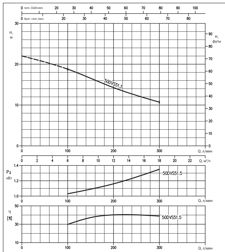
ГРАФИК РАБОЧИХ ХАРАКТЕРИСТИК (по ISO 9906, Приложение A)
