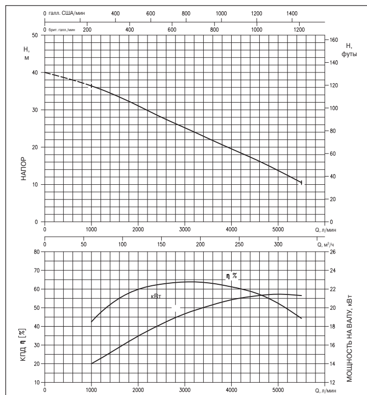
ГРАФИК РАБОЧИХ ХАРАКТЕРИСТИК серии 150DML522 (по ISO 9906, Приложение А) ДИАМЕТР РАБОЧЕГО КОЛЕСА: 330 мм
