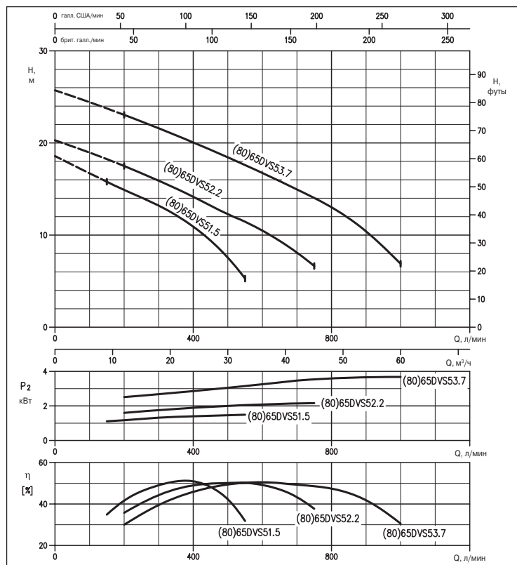
ГРАФИК РАБОЧИХ ХАРАКТЕРИСТИК (по ISO 9906, Приложение A)
