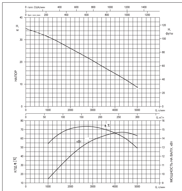
ГРАФИК РАБОЧИХ ХАРАКТЕРИСТИК серии 150DML 515 (по ISO 9906, Приложение А) ДИАМЕТР РАБОЧЕГО КОЛЕСА: 309 мм
