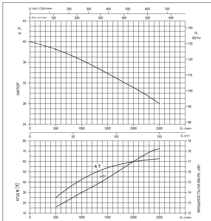
ГРАФИК РАБОЧИХ ХАРАКТЕРИСТИК серии 100DML522 (по ISO 9906, Приложение А) ДИАМЕТР РАБОЧЕГО КОЛЕСА: 330 мм
